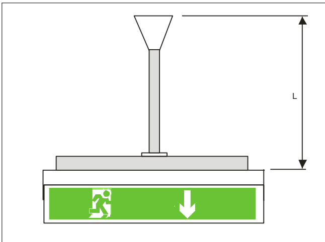
Pendelmontage
