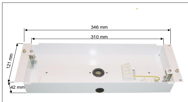
B-COV 8 - Boîtier d'encastement
